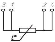
СХЕМА СОЕДИНЕНИЙ
